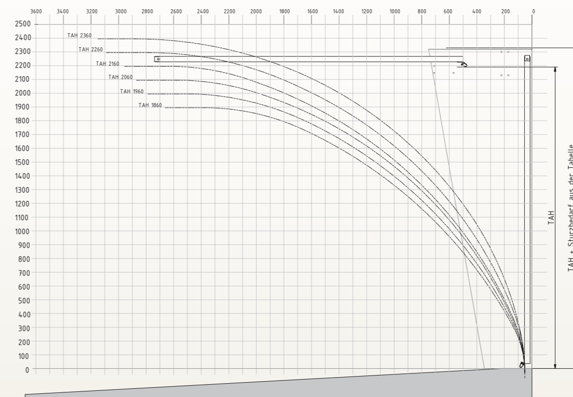
ÖFFNUNGSKURVE KEN 46
